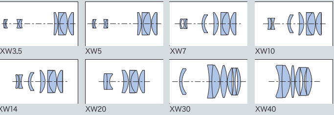
■XWシリーズレンズ構成図
