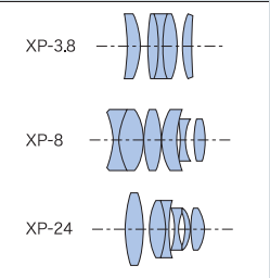
■XPシリーズレンズ構成図
