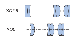
■XOシリーズレンズ構成図
